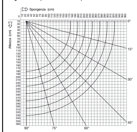
Diagramma di copertura - Installazione parete e soffitto
